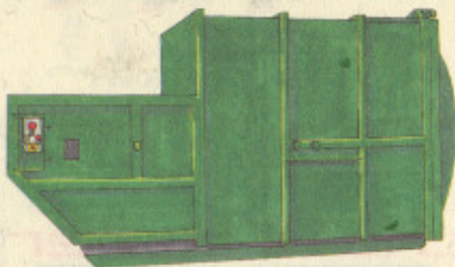
Selbstpresscontainer für Absetzkipper 10 cbm
